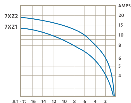
保護器廠的技術規格圖範例 1
